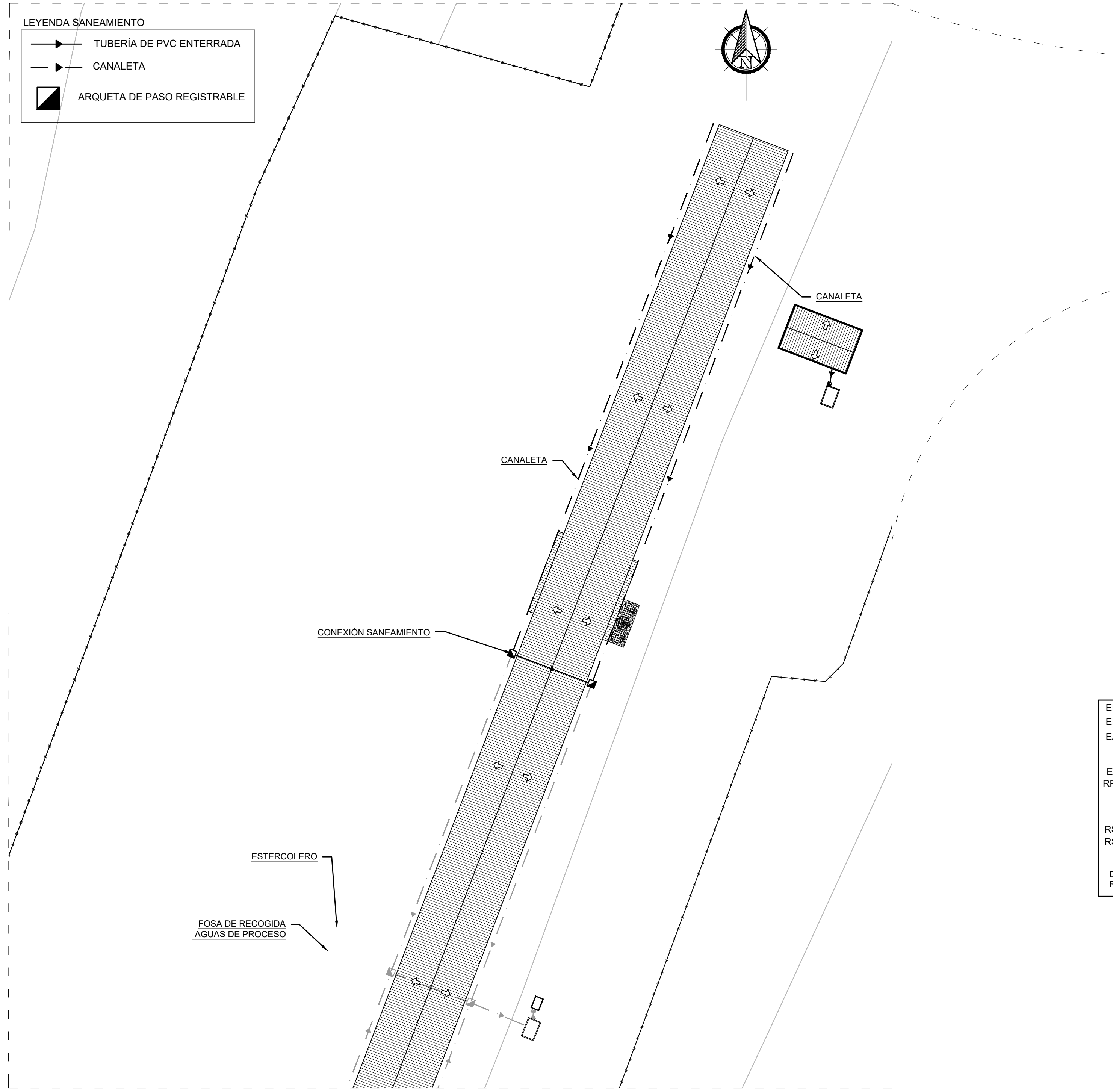
DISTRIBUCIÓN EN PARCELA Escala 1/500
