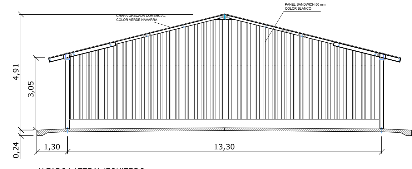
ALZADO LATERAL IZQUIERDO E 1/100
