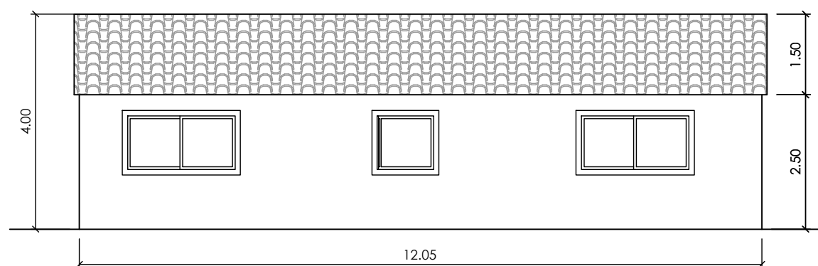
ALZADO LATERAL DE CASETA DE RIEGO Escala 1/100
