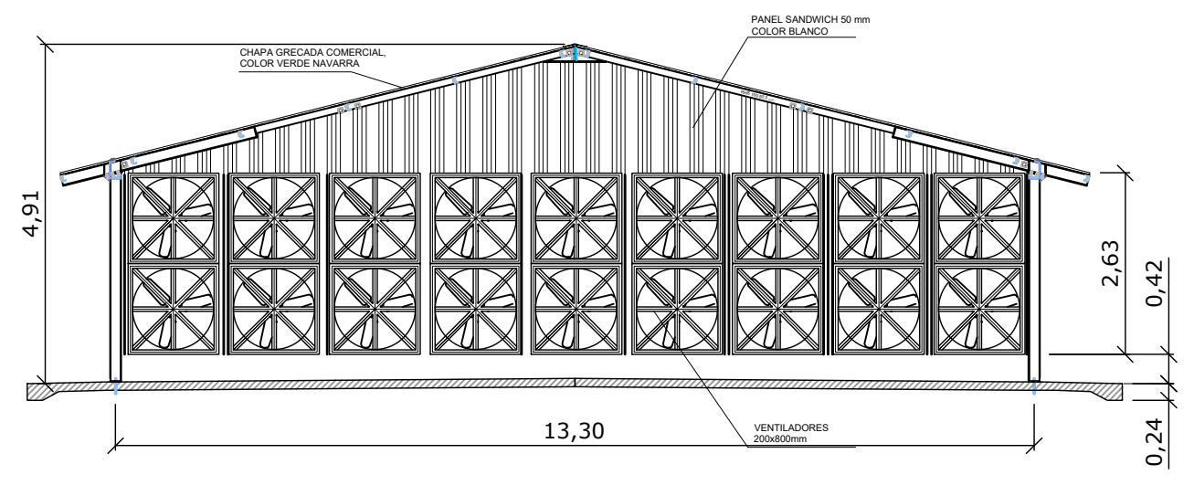
ALZADO LATERAL DERECHO E 1/100
